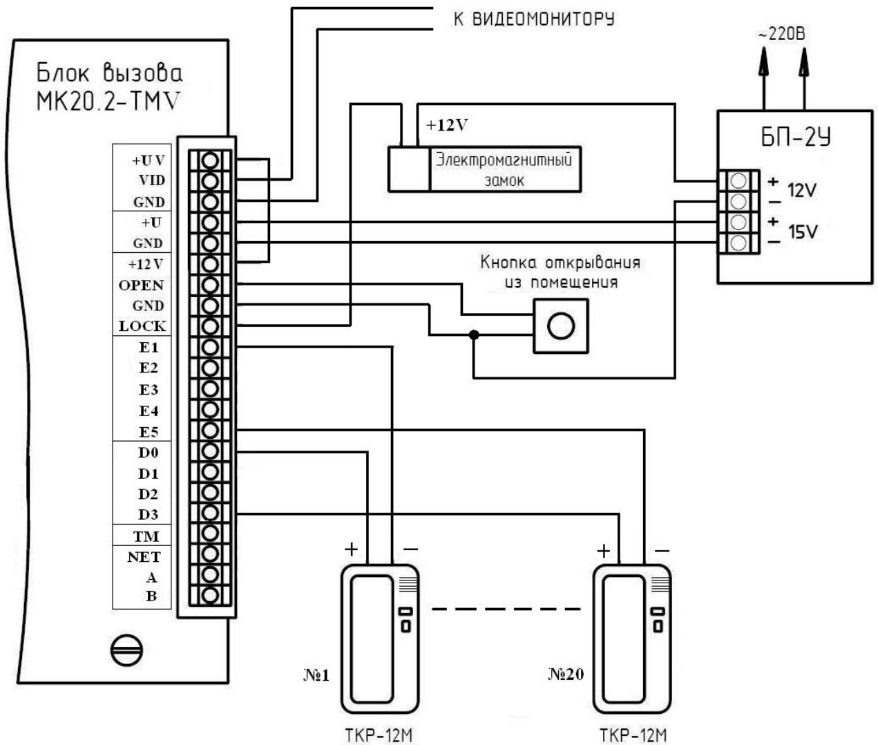
Рис. 2 Пример монтажа блока вызова МК20.2-ТМV
