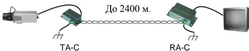
Рис.2 Схема подключения TA-C/1 и RA-C/1
