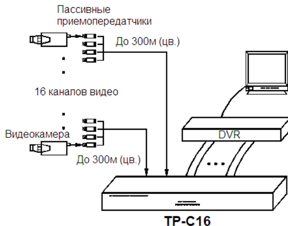
Рис.2 Схема подключения TP-C16
