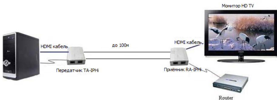
Рис.4 Схема подключения передатчика TA-IPHi и приемника RA-IPHi
