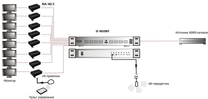
Рис. 4 Схема подключения разветвителя D-Hi108T (аналогично D-Hi104T)
