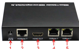
Рис. 4 Элементы приёмника HDBase-T.
