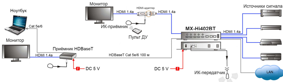
Рис. 5 Схема подключения коммутатора MX-Hi402BT.
