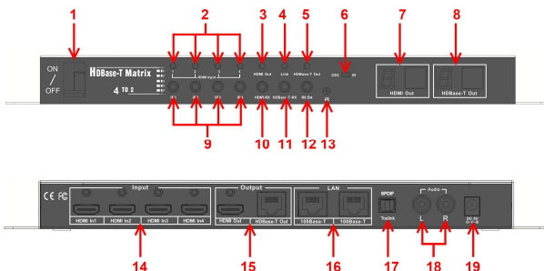
Рис. 3 Элементы коммутатора МХ-Нi402ВТ.
