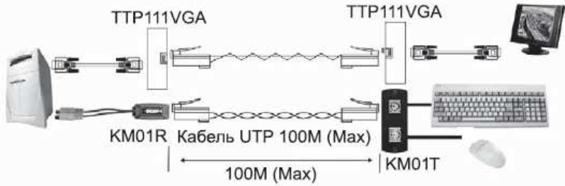
Рис. 3 Схема подключения КМ01, КМ02
