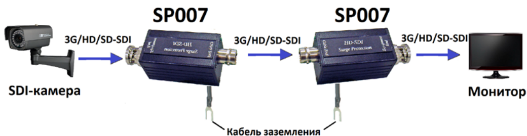
Рис.2 Схема подключения SP007.
