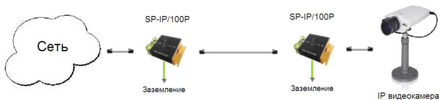
Рис.3 Подключение SP-IP/100P
